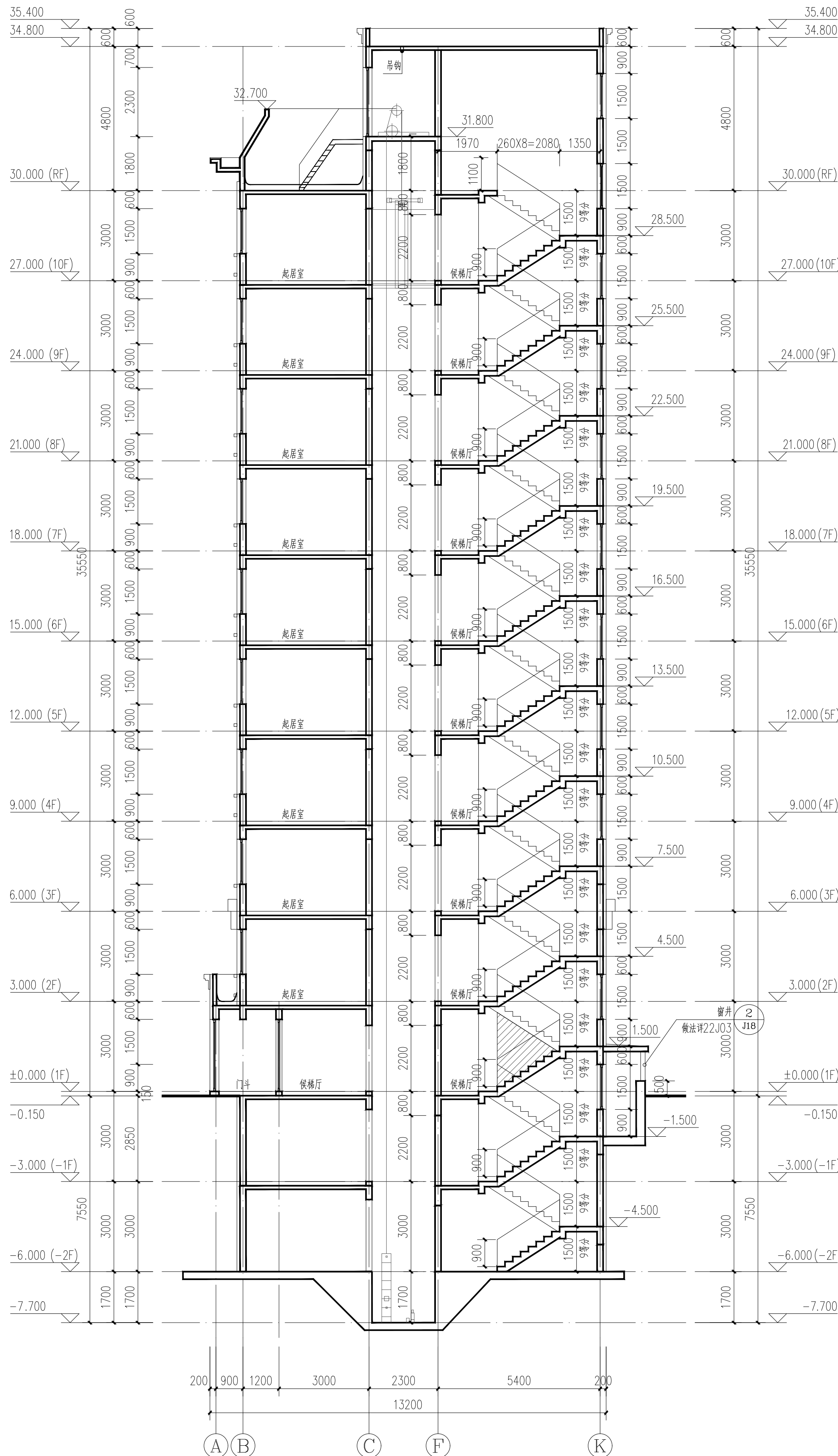
1-1剖面图 1:100
